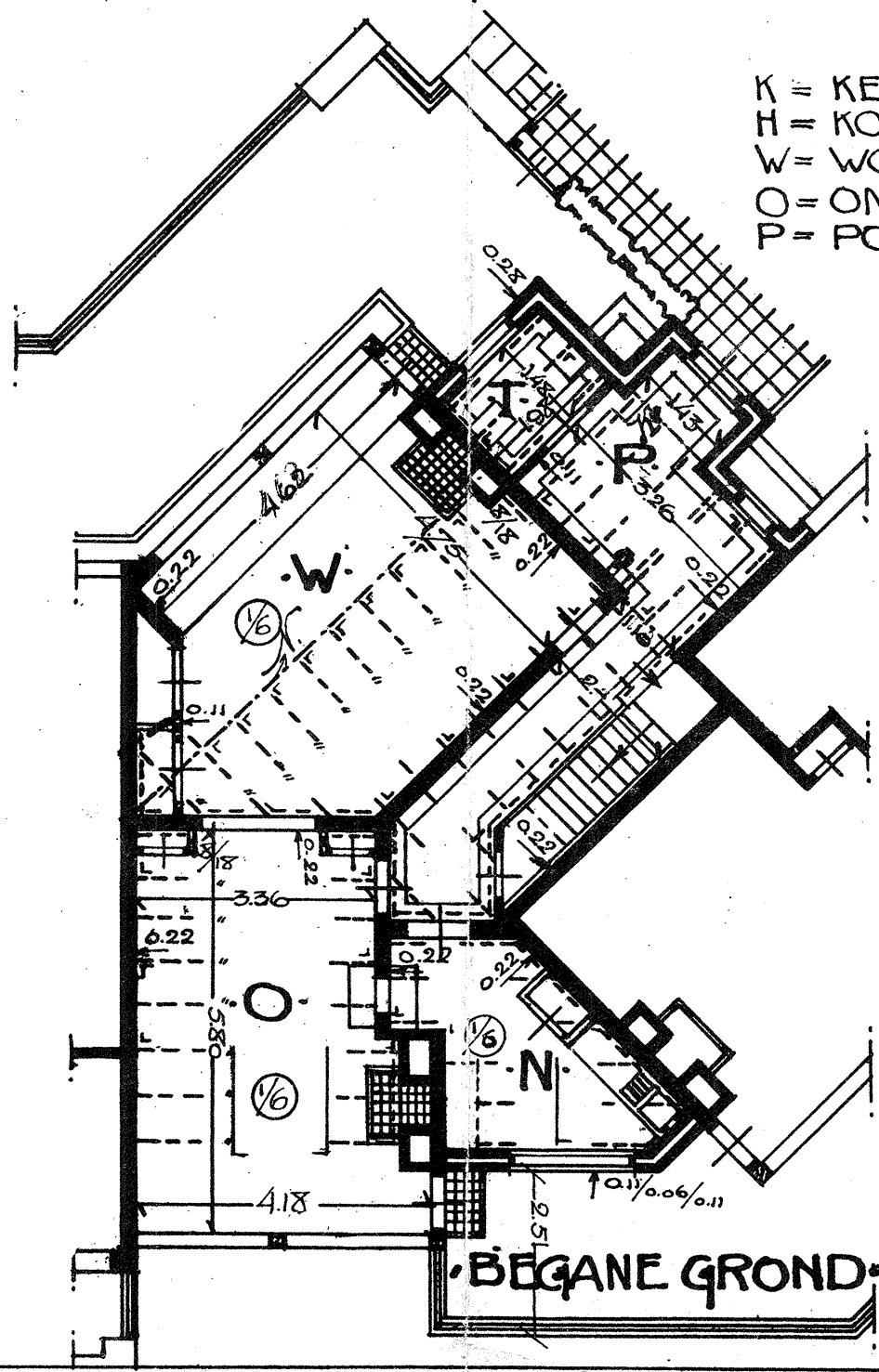
BEGANE GROND
