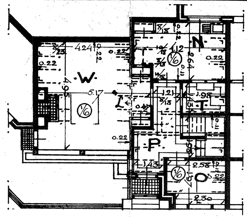
BEGANE GROND
