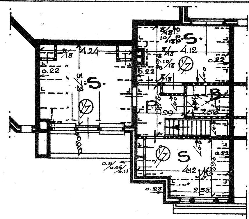
VERDIEPING
