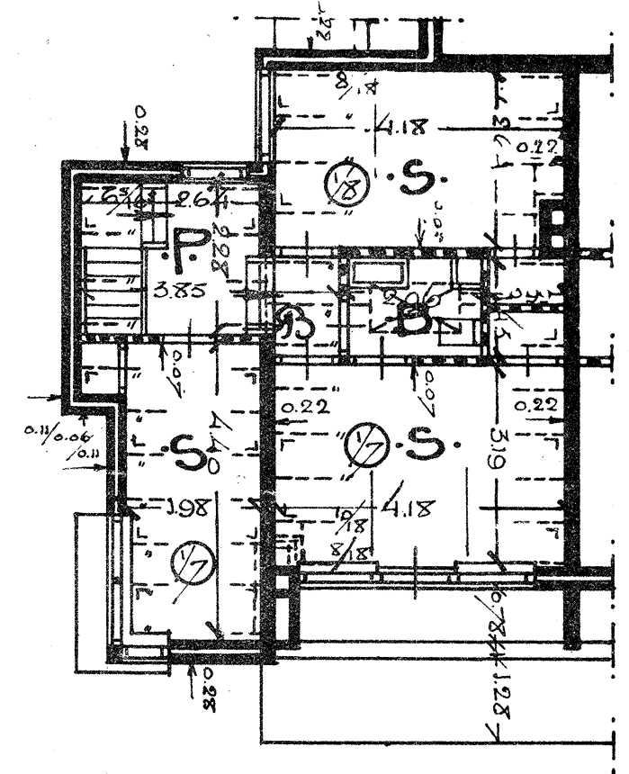
VERDIEPING
