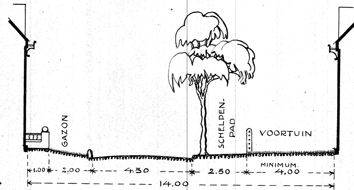
NORMAAL STRAATPROFIEL SCHAAL 1:100
