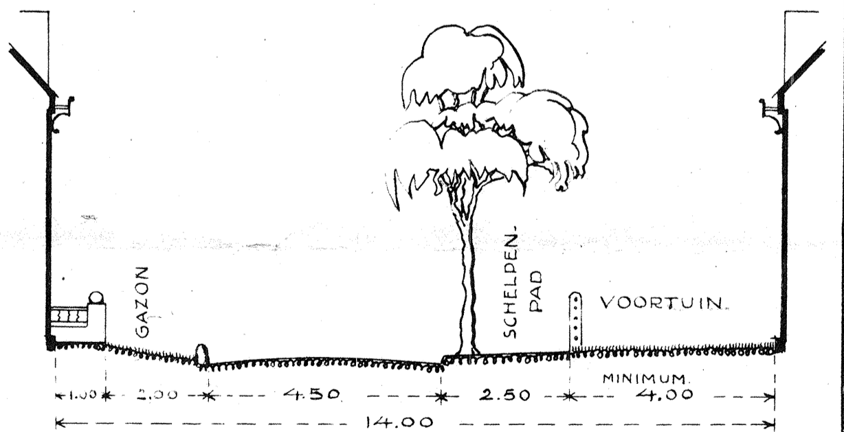
NORMAAL STRAATPROFIEL SCHAAL 1:100
