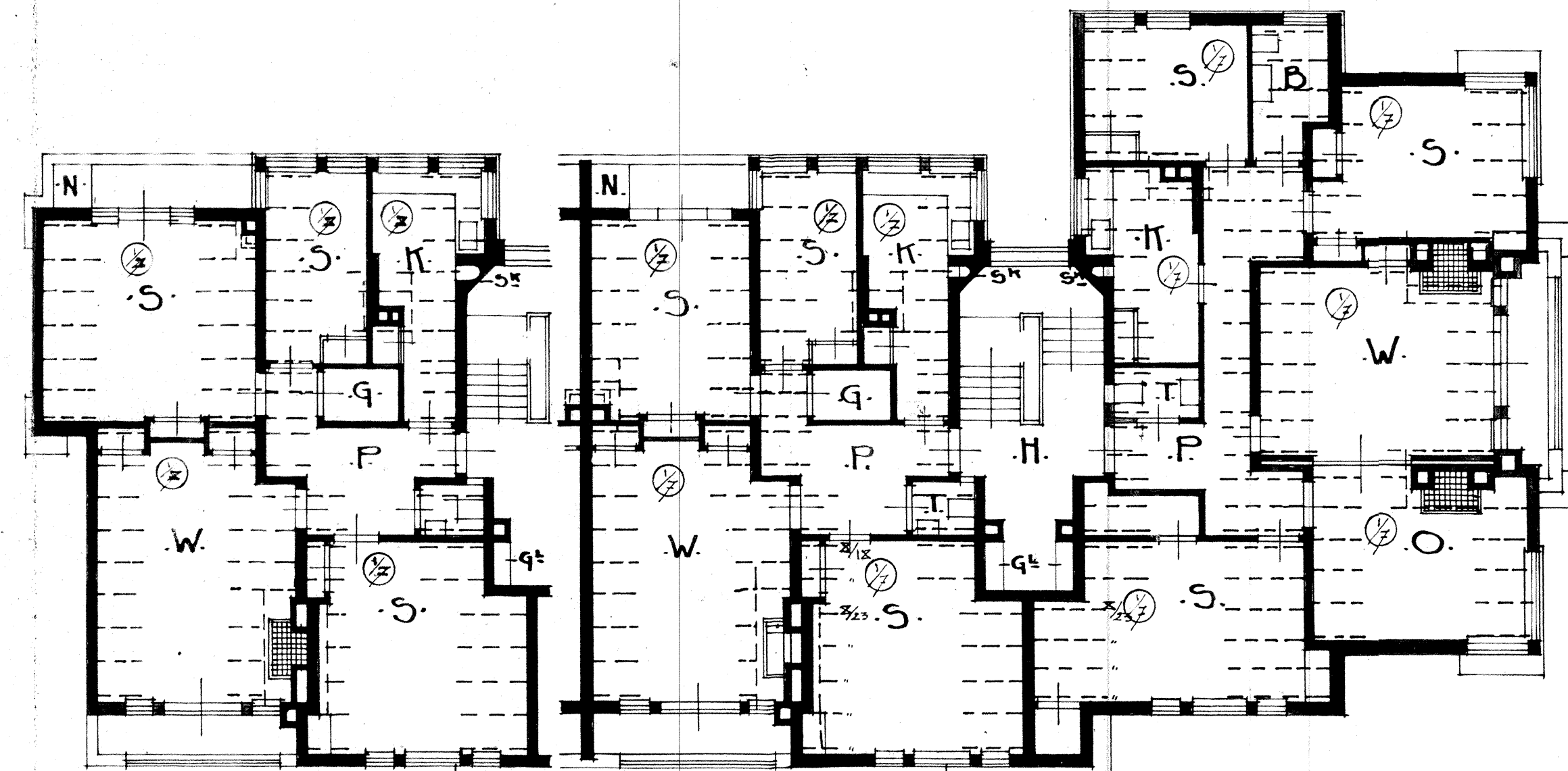
•EERSTE VERDIEPING• BALKZWARFEN ALSBOVEN BEG. GROND.
