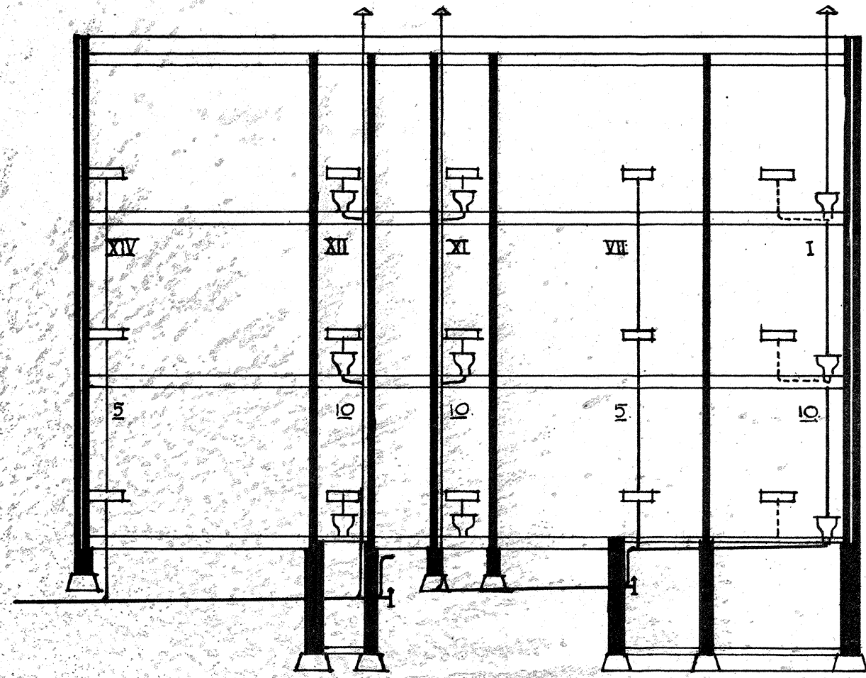
'DOORSNEDE A-B'
