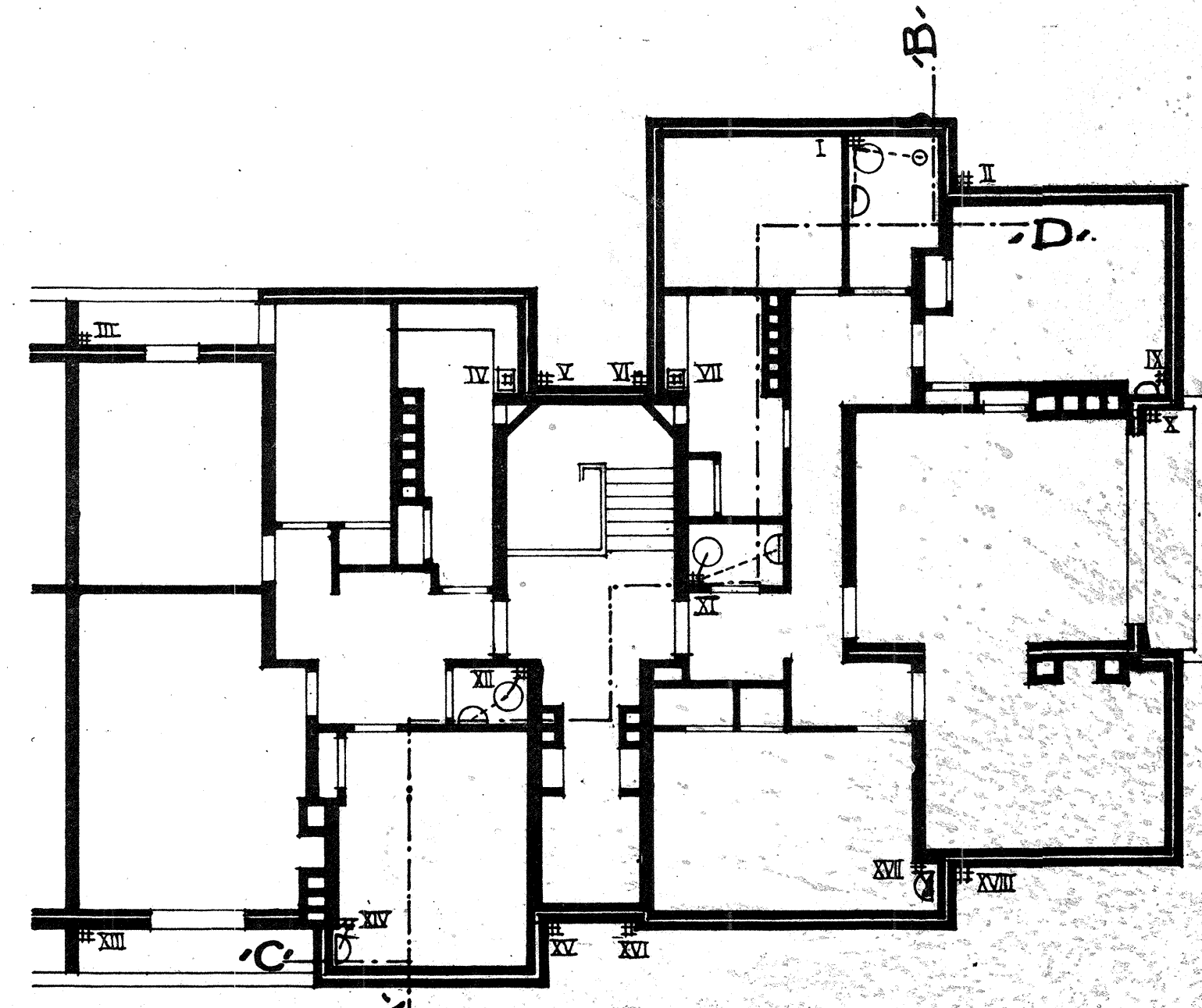
'TWEDE VERDIEPING'
